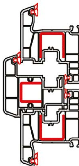
SISTEM PROZORA ŠTULP
