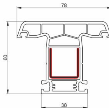
PVC PROFIL T PREČKA BW 6021
