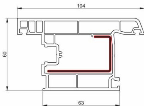
PVC PROFIL KRILO VRATA VANJSKO OTVARANJE BW 6051
