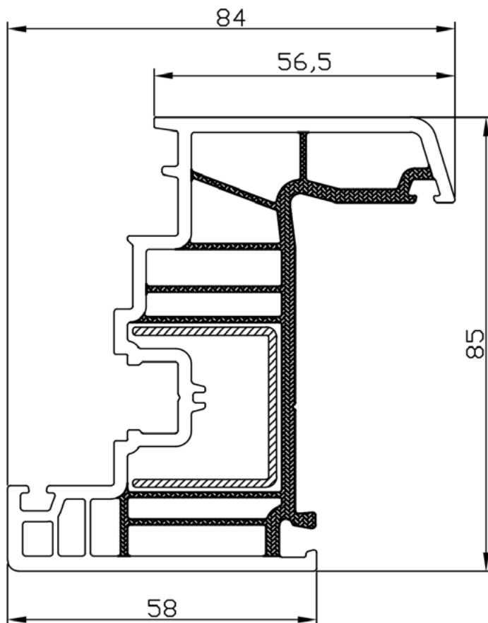
PVC PROFIL KRILO PROZORA BF 8512
