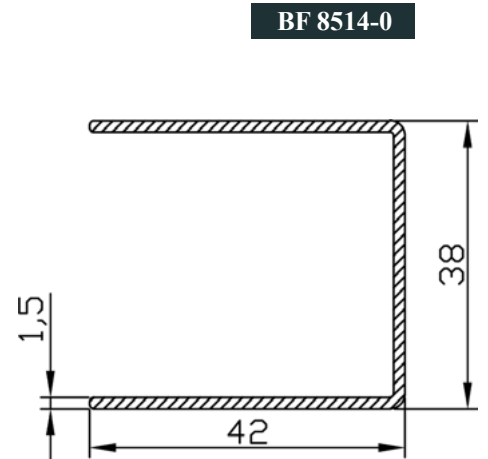
ŽELJEZNO OJAČANJE BF 8514-0
