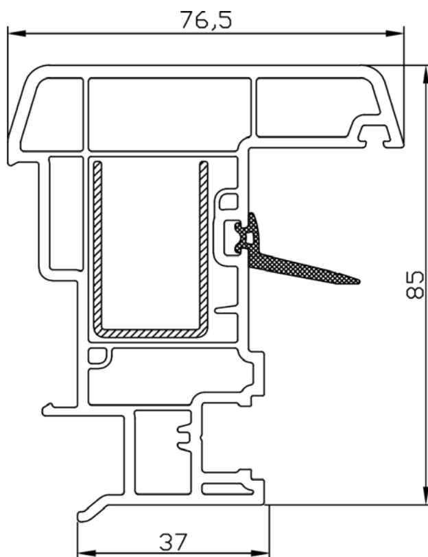
PVC PROFIL ŠTULP BF 8516
