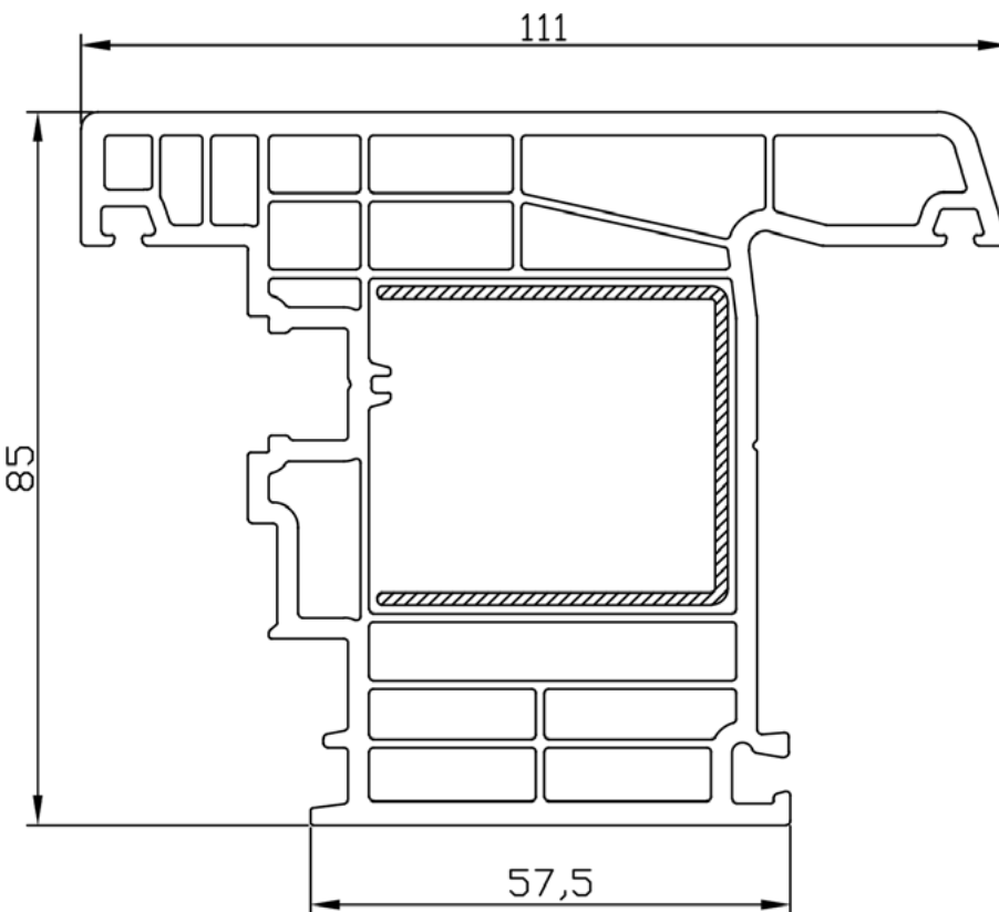
PVC PROFIL KRILO VRATA VANJSKO OTVARANJE BF 8514
