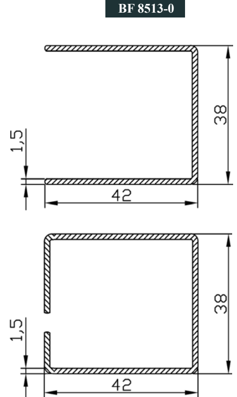
ŽELJEZNO OJAČANJE BF 8513-0
