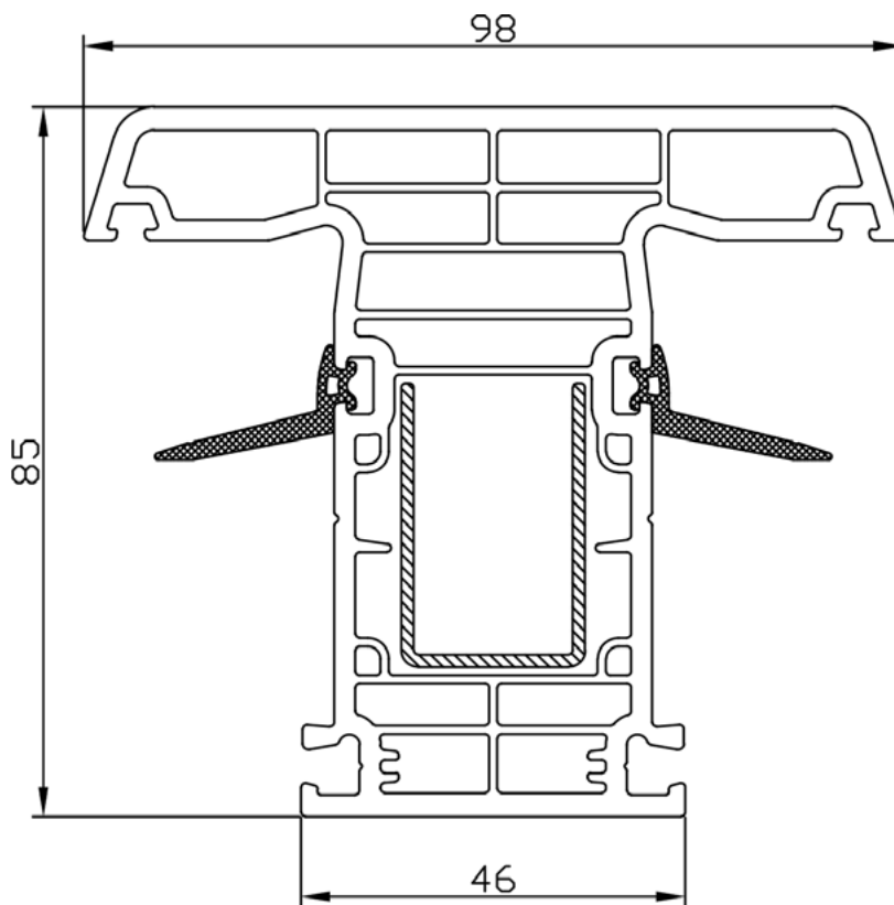
PVC PROFIL T PREČKA BF 8515
