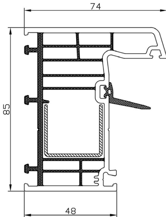
PVC PROFIL ŠTOKA BF 8511
