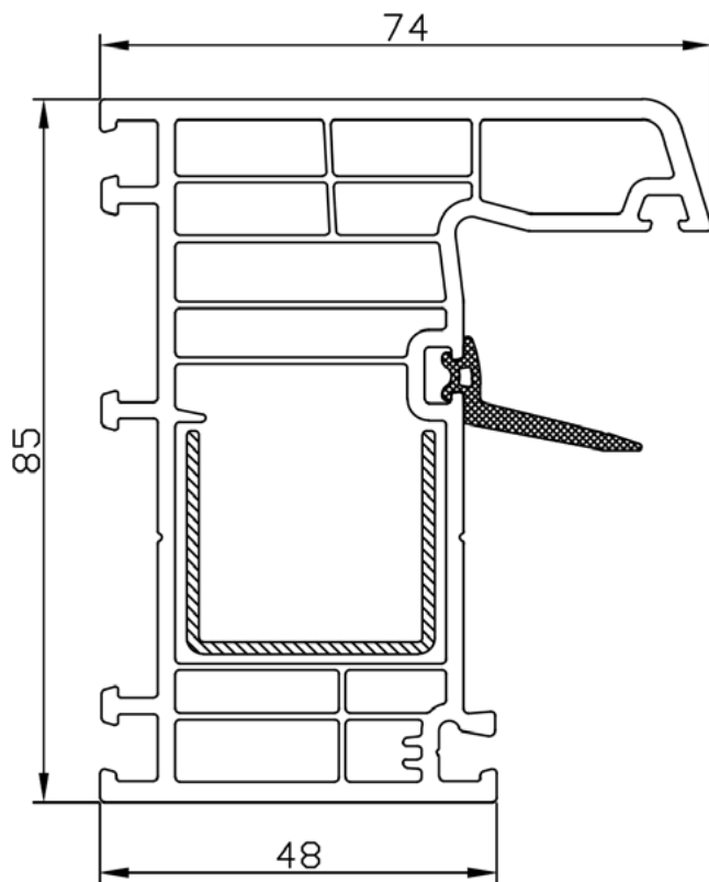
PVC PROFIL ŠTOKA BF 8501
