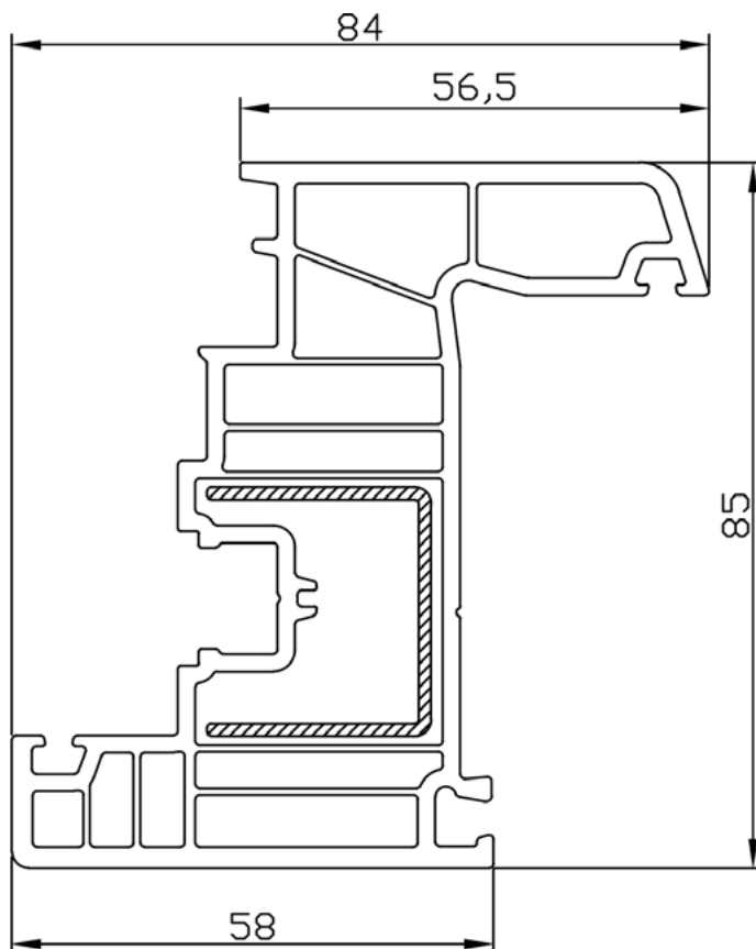
PVC PROFIL KRILO PROZORA BF 8502
