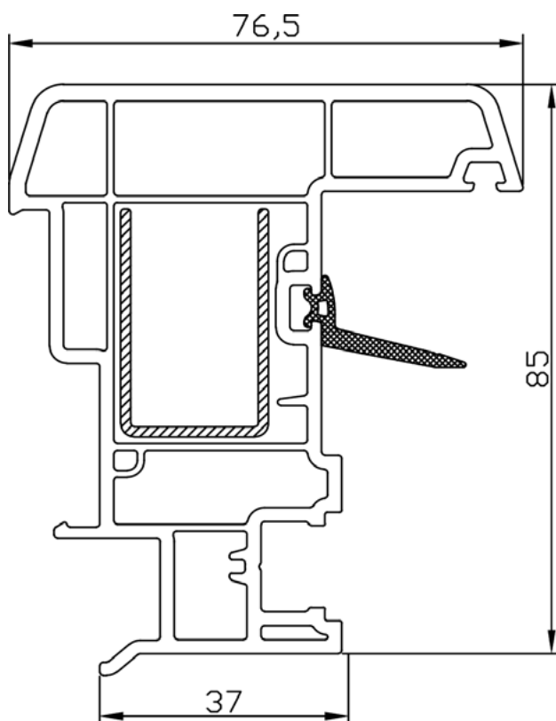
PVC PROFIL ŠTULP BF 8506
