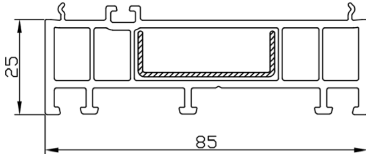
PVC PROFIL PROŠIRENJE BF 8507
