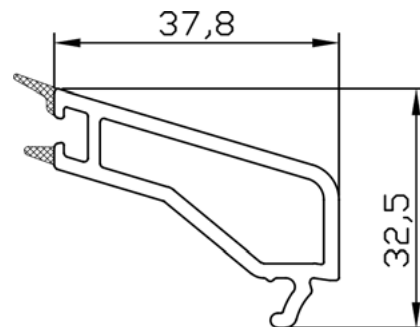
PVC LAJSNA BF 8509
