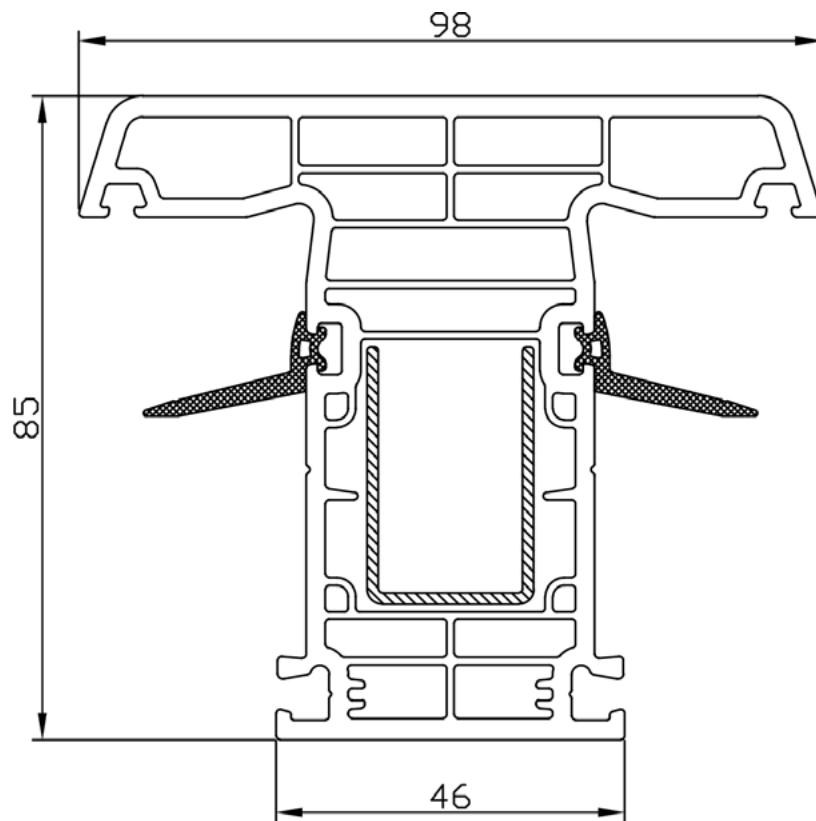
PVC PROFIL T PREČKA BF 8505
