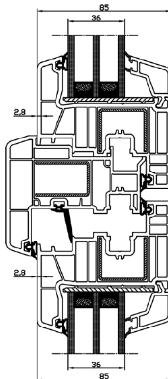
SISTEM PROZORA ŠTULP
