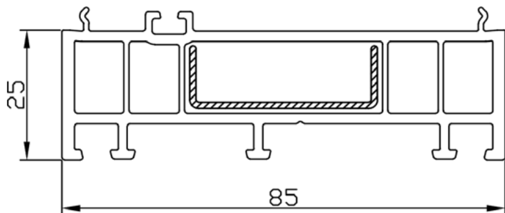
PVC PROFIL PROŠIRENJE BF 8507
