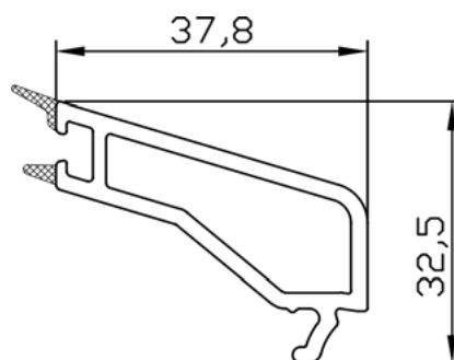
PVC LAJSNA BF 8509
