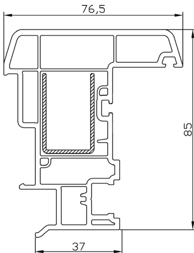
PVC PROFIL ŠTULP BF 8526
