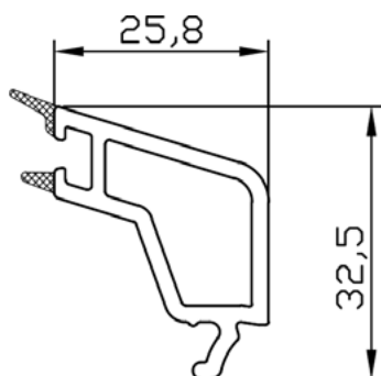
PVC LAJSNA BF 8508
