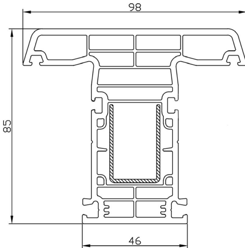
PVC PROFIL T PREČKA BF 8525
