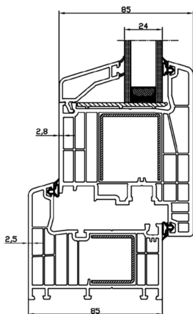
SISTEM VRATA VANJSKO OTVARANJE
