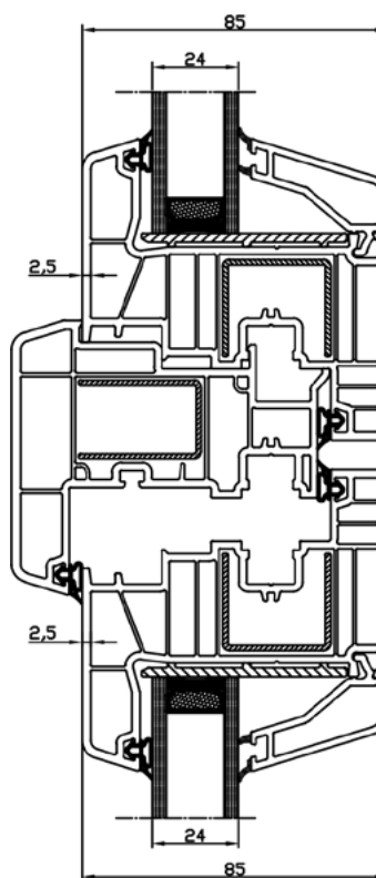
SISTEM PROZORA ŠTULP
