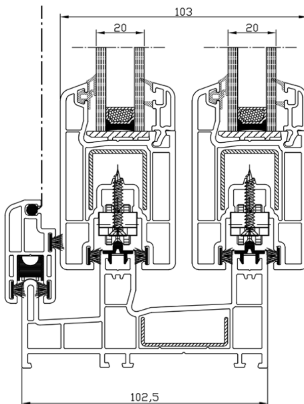
KLIZNI SISTEM SA KOMARNIKOM
