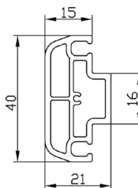
PVC PROFIL PREČKE SA KOMARNIKOM
