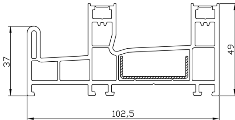
PVC PROFIL ŠTOKA SA KOMARNIKOM
