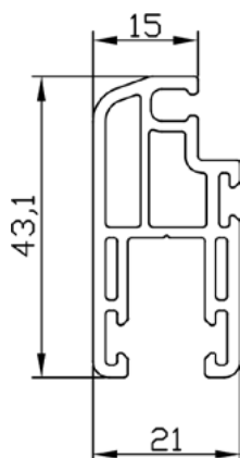
PVC PROFIL KRILA SA KOMARNIKOM
