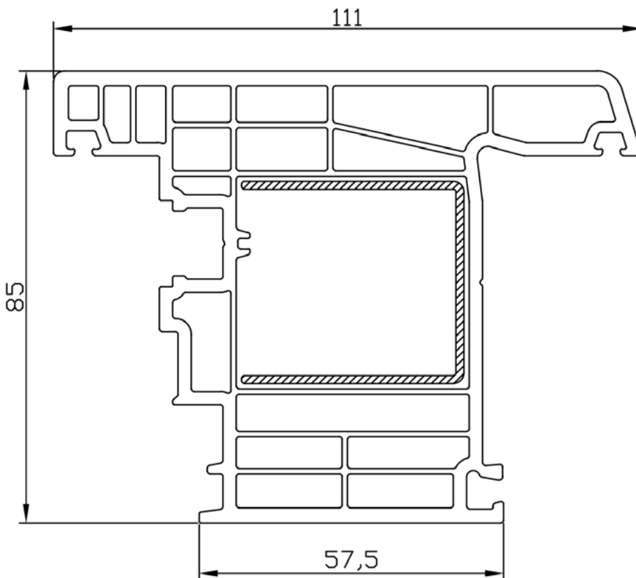
PVC PROFIL KRILO VRATA BF 8514 VANJSKO OTVARANJE
