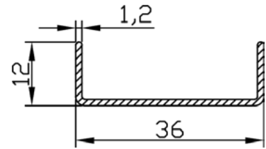
ŽELJEZNO OJAČANJE BF 8507-0
