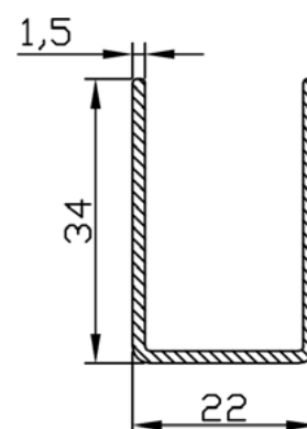
ŽELJEZNO OJAČANJE BF 8526-0
