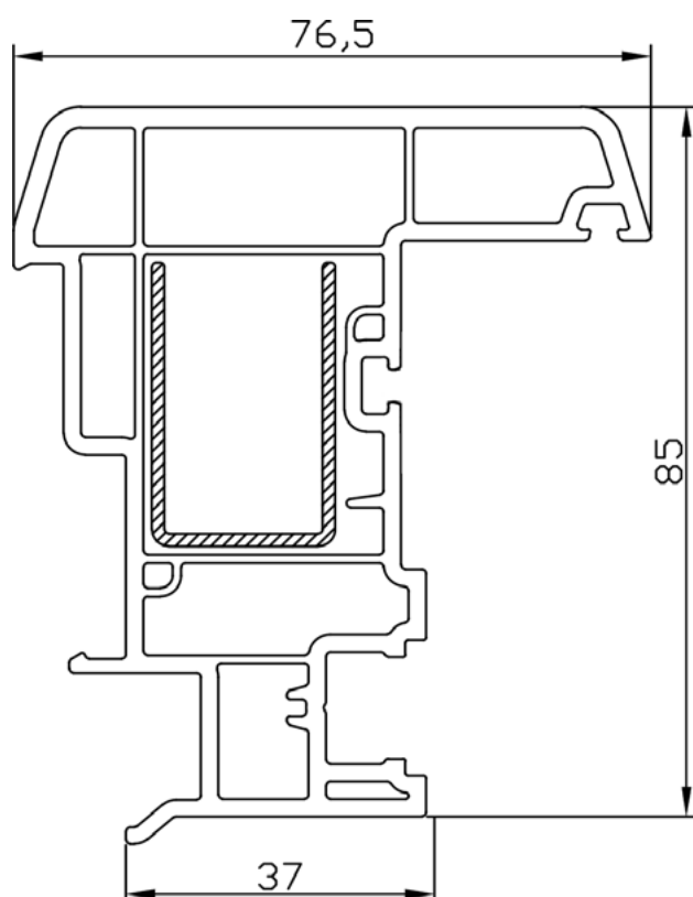
PVC PROFIL ŠTULP BF 8526
