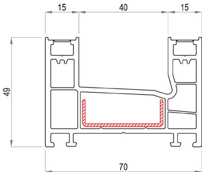
PVC PROFIL ŠTOKA BW 9001
