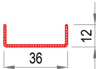
PVC PROFIL ŠTULP BW 6001
