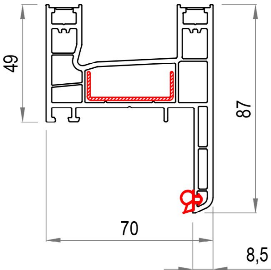
PVC PROFIL ŠTULP BW 6001
